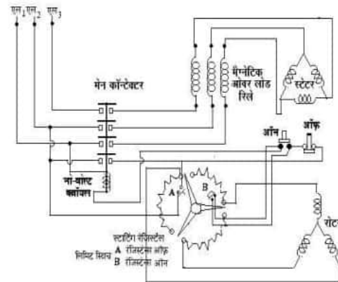
रजिस्टर्स टाइम रिले रिंग मोटर स्टार्टर का कनेक्शन डायग्राम
