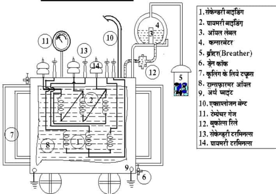
ट्रान्सफार्मर के विभिन्न भाग
