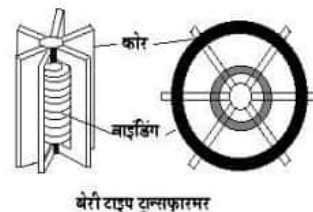
बेरी टाइप ट्रांसफार्मर
