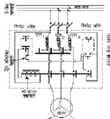
डायरेक्ट ऑन-लाइन स्टार्टर का चित्र
